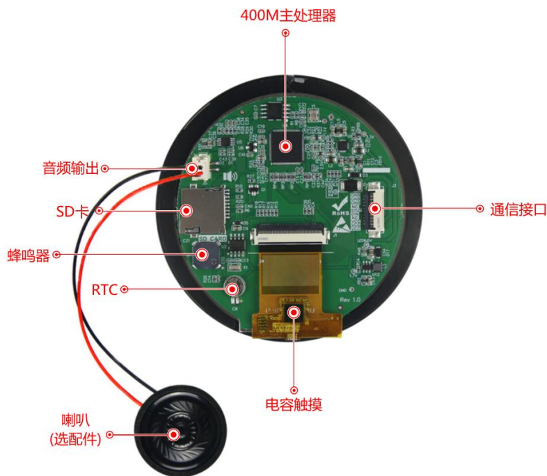
图 1-2 硬件配置图
